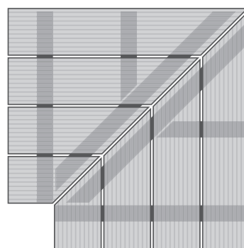
примерное расположение лаг для досок, обрезанных под углом 45°
