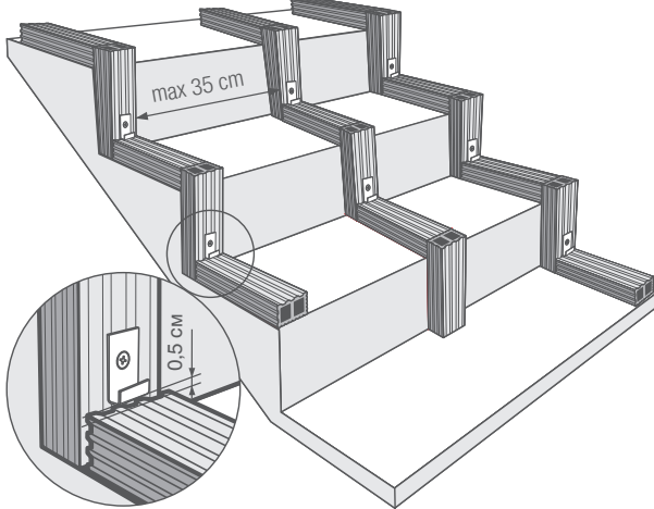
монтаж лаг и стартовых клипс на ступенях
