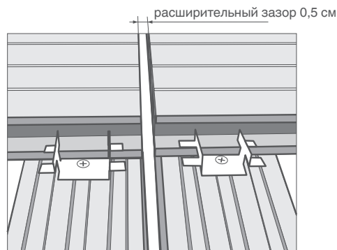
торцевое соединение досок на двух лагах
