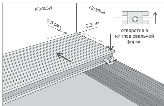
монтаж первой доски с помощью монтажной клипсы
