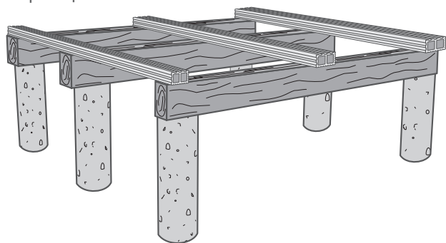
основание на грунте - терраса на бетонных опорах и деревянных лагах, более прочных, чем лаги из ДПК
