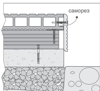
монтаж планки с помощью саморезов
