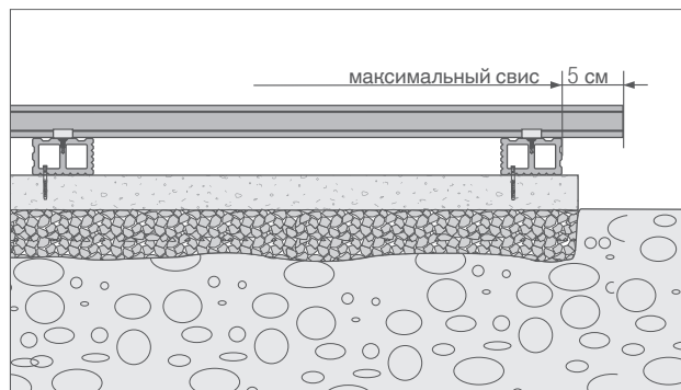
максимальный выступ доски за край лаги 5 см
