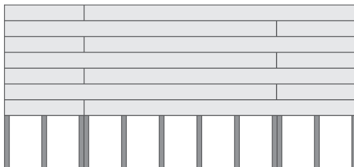
расположение лаг при торцевом соединении досок – терраса в так наз. «шахматном порядке»
