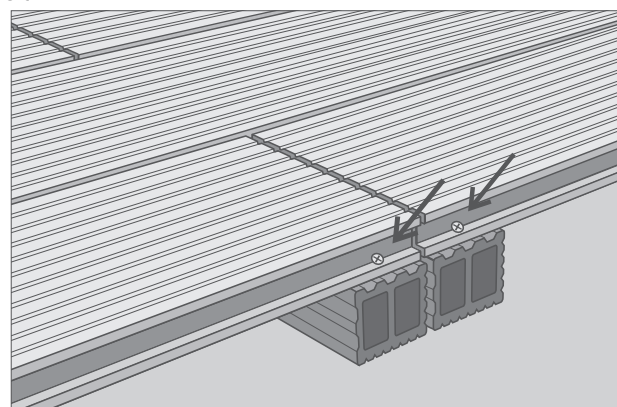
монтаж последних досок с помощью саморезов под углом
