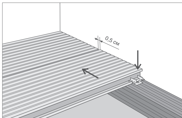
монтаж очередной доски с помощью монтажной клипсы
