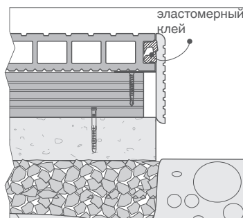
монтаж планки с помощью эластомерного клея
