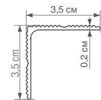
угловая алюминиевая декоративная планка
