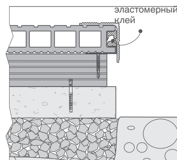
монтаж планки с помощью эластомерного клея
