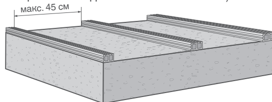
бетонное основание - терраса на бетонном основании
