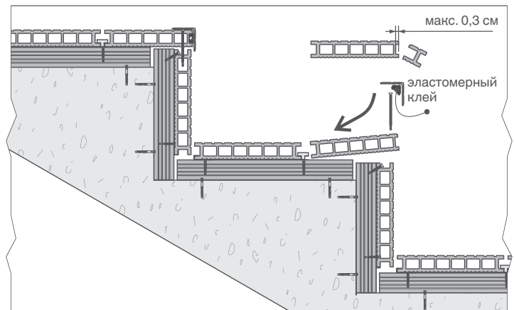
крепление горизонтальных досок обрезка и монтаж с угловой планкой
