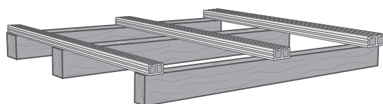
лаги на деревянной конструкции
