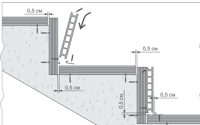
dylatacja czołowa między legarami, dylatacja klipsów do powierzchni prostopadłych, montaż desek i klipsów startowych na schodach
