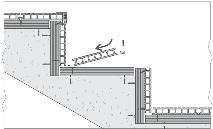
крепление горизонтальных досок
