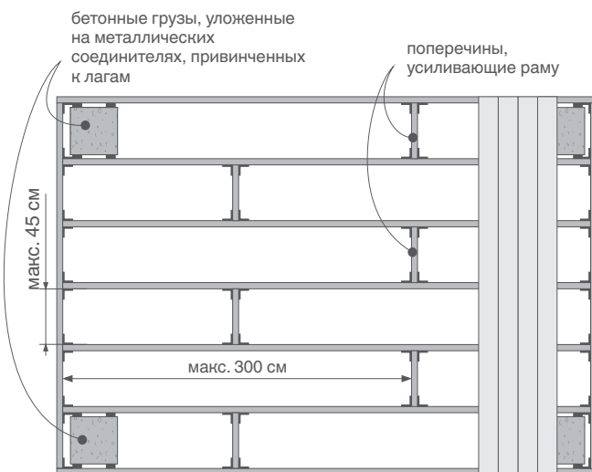
плавающая терраса - рама из лаг, соединенная при помощи металлических соединителей, нагруженная бетонными плитами
