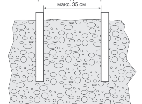
основание на грунте - терраса на бетонных опорах
