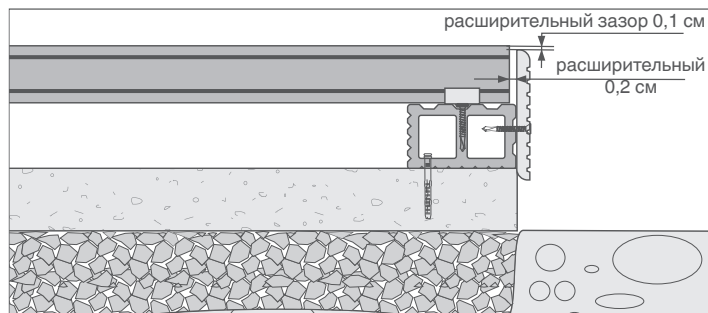
расширительный зазор 0,2 см между композитной декоративной планкой и торцевой поверхностью доски
