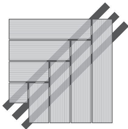
примерное расположение лаг для досок, уложенных «елочкой»
