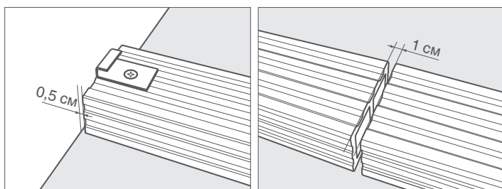
расположение лаг при торцевом соединении досок – терраса в так наз. «шахматном порядке»
