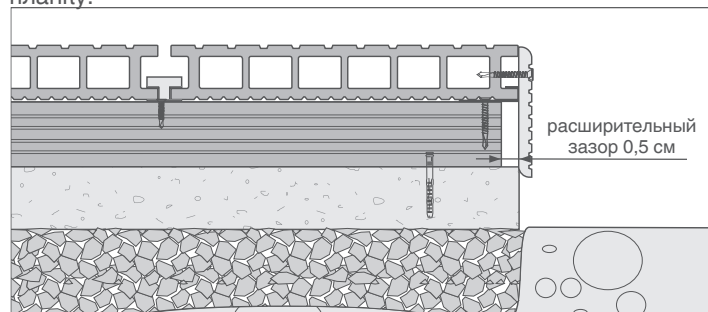
расширительный зазор 0,5 см между композитной декоративной планкой и торцевой поверхностью лаги
