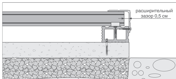
расширительный зазор 0,5 см между композитной декоративной планкой и торцевой поверхностью доски
