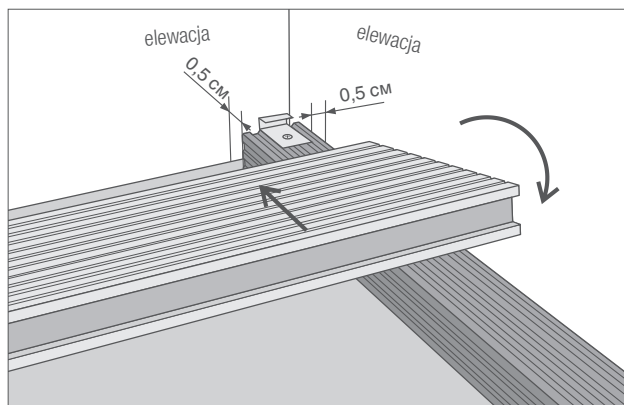
монтаж первой доски с помощью стартовой клипсы
