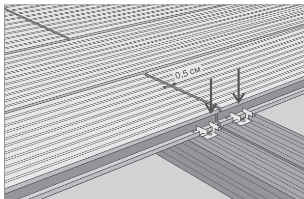
торцевое соединение досок на двух отдельных лагах (расширительный шов 0,5 см)
