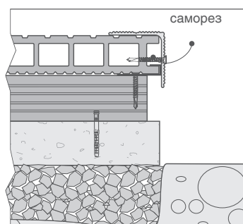
монтаж планки с помощью саморезов
